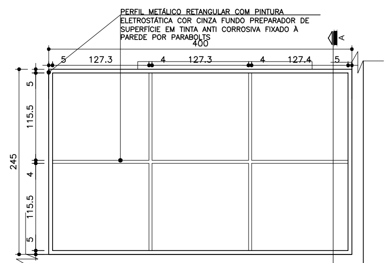
04 Planta Estrutura Metálica-Marquise Sala de Atividades Esc.: 1:50
